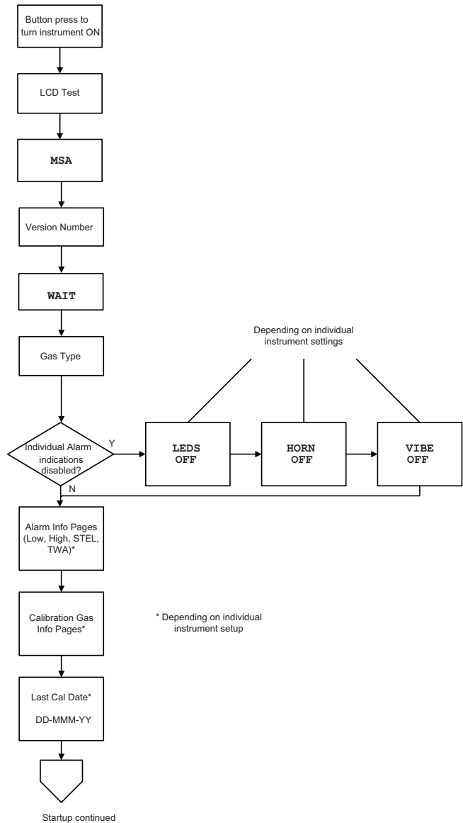
Fig. 3 Startup
